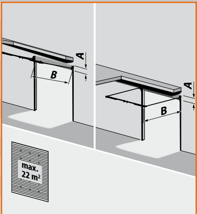
T 340, normaal railsysteem, verenpakket achter + stalen draagprofiel A= 340 mm B= daghoogte + 750 mm Breedte max. 6.500 mm
