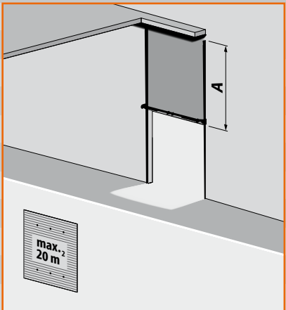
T 500 hF, verticaal railsysteem met laagliggende veeras + stalen draagprofiel A= daghoogte + 400 mm, Breedte max. 4.500 mm
