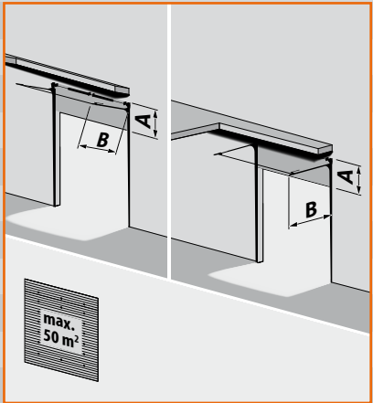
T 400, verhoogd railsysteem A= heffing + 400 mm B= daghoogte – heffing + 600 mm
