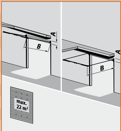
T 240, laagbouw railsysteem, binnenliggende kabels + stalen draagprofiel A= 240 mm B= daghoogte + 1.000 mm Breedte max. 6.500 mm
