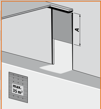
T 500, verticaal railsysteem A= daghoogte + 560 mm
