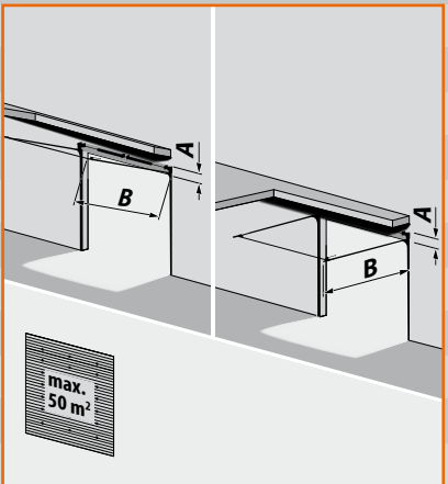
T 450, normaal railsysteem (standaard) A = 430-510 mm B= daghoogte + 650 mm
