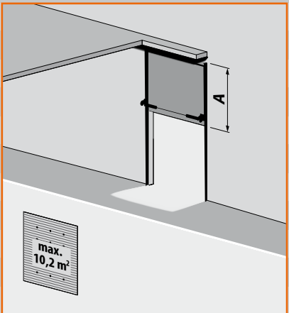
T500 DS verticaal railsysteem met laagliggende veeras A= daghoogte + 400 mm Breedte max. 3.200 mm Hoogte max. 3.200 mm
