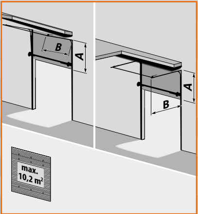
T400 DS verhoogd railsysteem met laagliggende veeras A= heffing + 200 mm B= daghoogte – heffing + 600 mm Breedte max. 3.200 mm Hoogte max. 3.200 mm Heffing min. 1.700 mm
