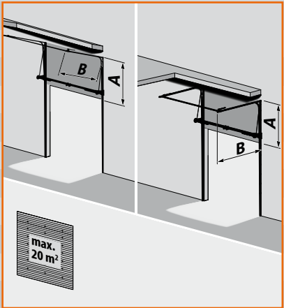
T 400 hF, verhoogd railsysteem met laagliggende veeras + stalen draagprofiel A= heffing + 200 mm B= daghoogte – heffing + 600 mm Breedte max. 4.500 mm Heffing min. 1.450 mm
